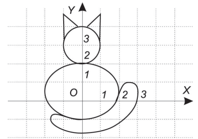
Рис. 1♦1. Комплексная кошка.
